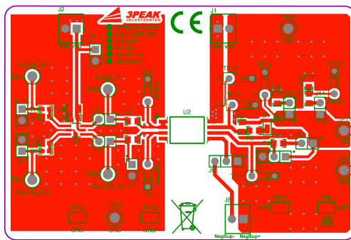
Top Layer
