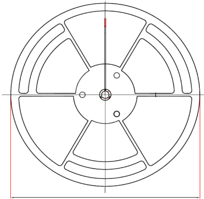
D1: Reel Diameter
